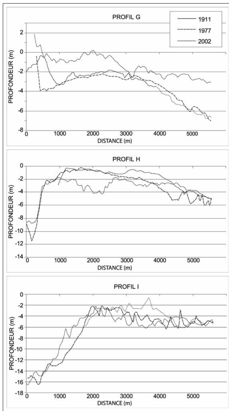
Fig. 9 – Evolution des profils bathymétriques longitudinaux de 1911 à 2002 (voir la fig. 4 pour la localisation des profils G à I).
