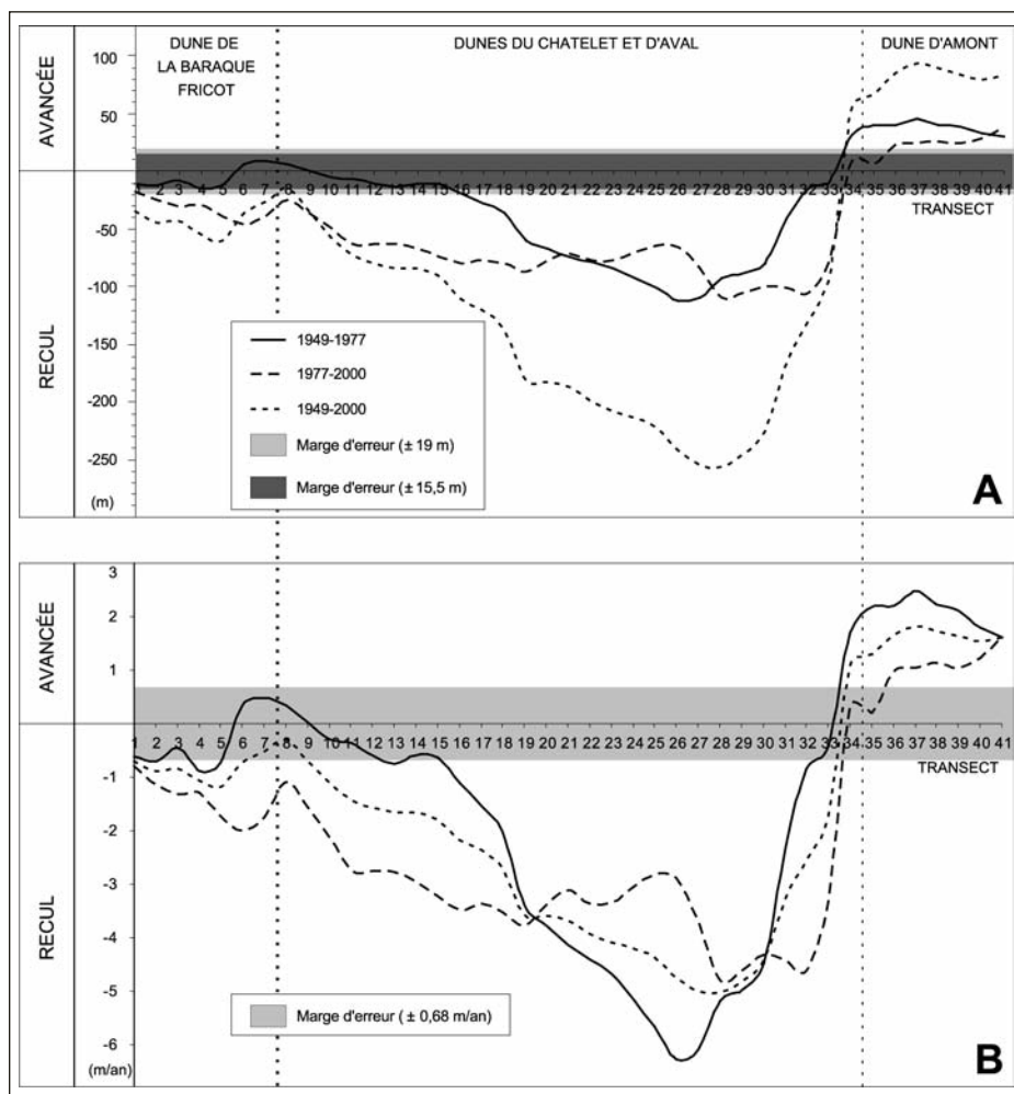
Fig. 6 – A) : évolution de la position du trait de côte en Baie de Wissant entre 1949 et 2000 ; B) : rythmes annuels d'évolution du trait de côte pour les périodes 1949-1977, 1977-2000, et 1949-2000.
