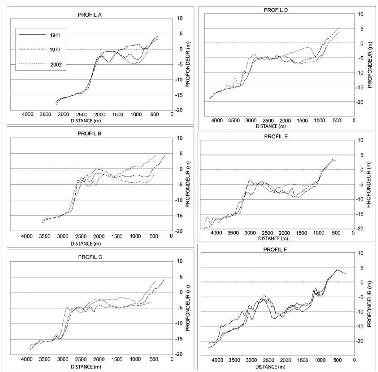
Fig. 8 – Evolution des profils bathymétriques transversaux de 1911 à 2002 (voir la fig. 4 pour la localisation des profils A à F).
