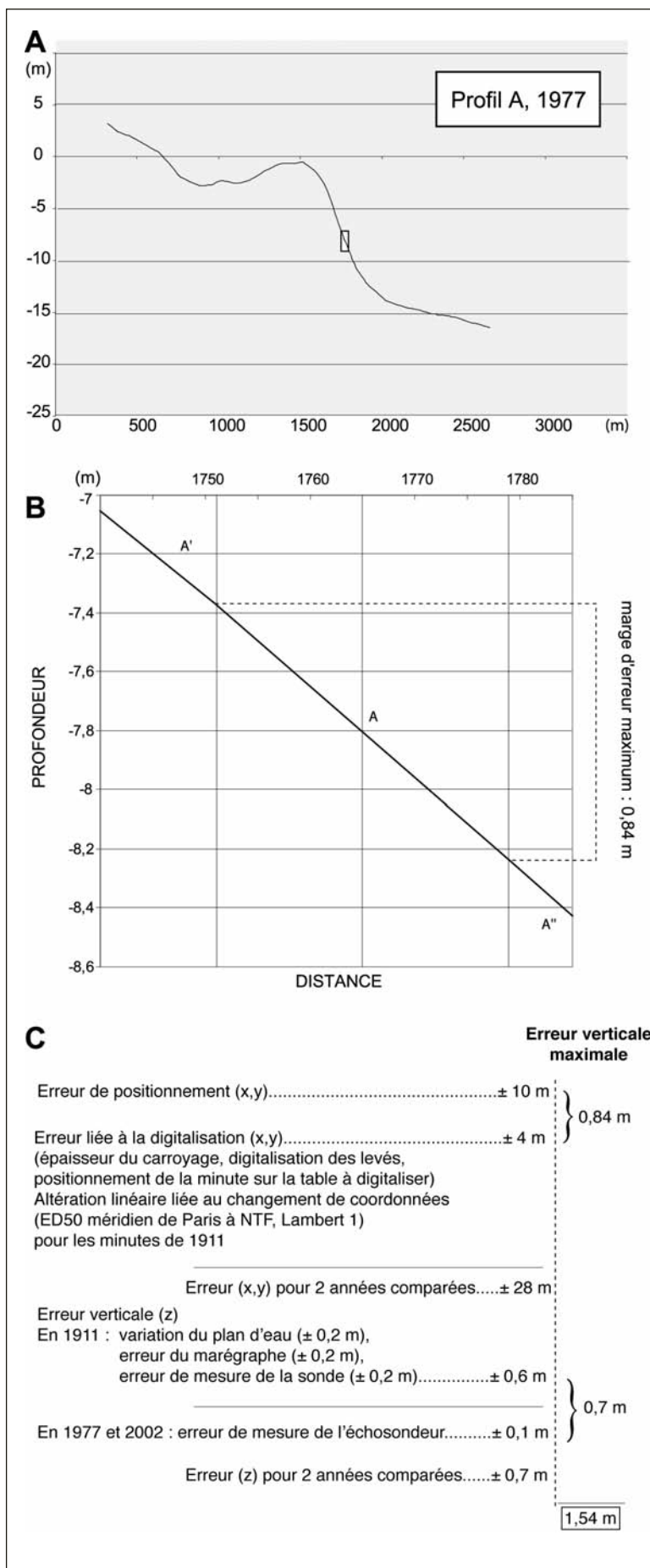
Fig. 5 – Estimation de la marge d'erreur des données bathymétriques. A) et B) : exemple de détermination de l'erreur verticale maximale pouvant être induite par une erreur de positionnement sur une pente sous-marine ; C) : détermination de la marge d'erreur totale.
