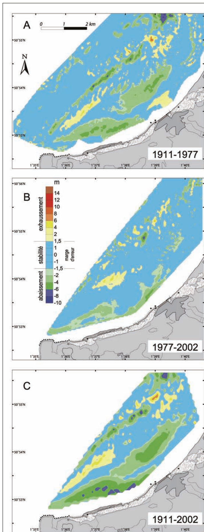
Fig. 7 – Cartes d'évolution de la bathymétrie en baie de Wissant pour les périodes (A) 1911-1977, (B) 1977-2002, et (C) 1911-2002 (données SHOM 2001, contrat n° E70/2001).
